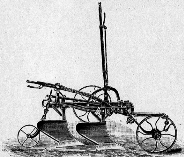
Brandenburger Completpflug mit Lenksteuer zur Arbeit eingestellt.
