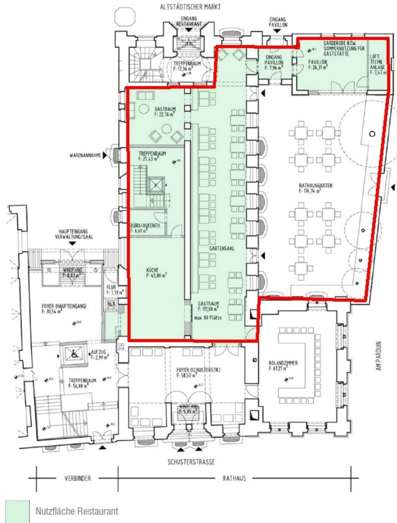
Altstädtisches Rathaus Grundriss Erdgeschoss M 1:200
