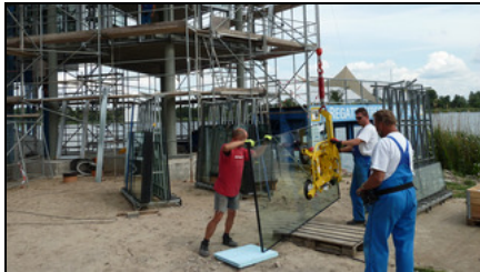
Moderne Technik hilft beim Einsetzen der großen Glasscheiben für die Fensterfronten.
